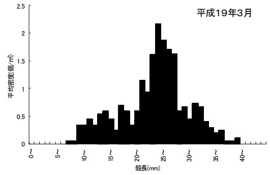
図7 吉富干潟におけるアサリ分布密度
