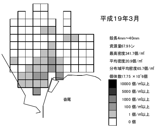
図4 沓尾干潟におけるアサリ分布密度
