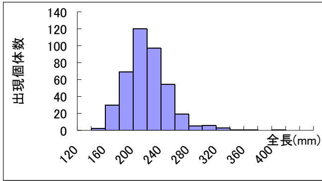
図3 マコガレイの市場における全長組成
