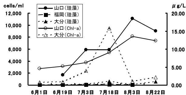
図12 全珪藻類細胞数とクロフィル量の推移 (全層平均)
