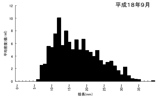
図4 沓尾干潟におけるアサリ分布密度
