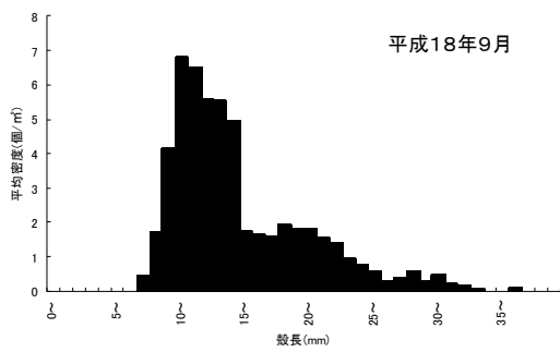
図2 蕨島干潟におけるアサリ分布密度
