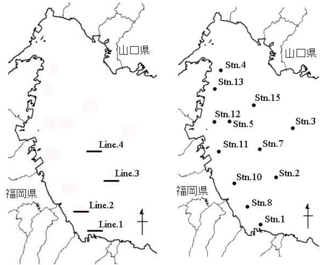
図1 調査地点（左：調査定線 右：浅海定線調査点）
