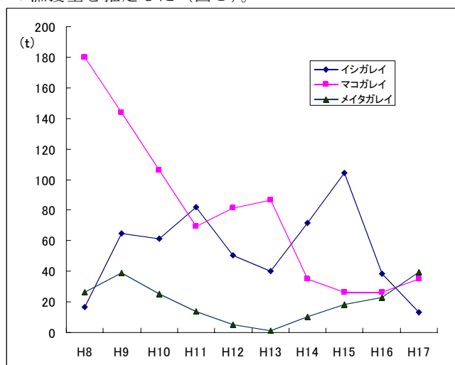
図1 カレイ類の漁獲量の推移
