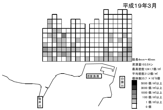
図6 吉富干潟におけるアサリ分布密度
