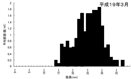
図5 沓尾干潟におけるアサリ分布密度
