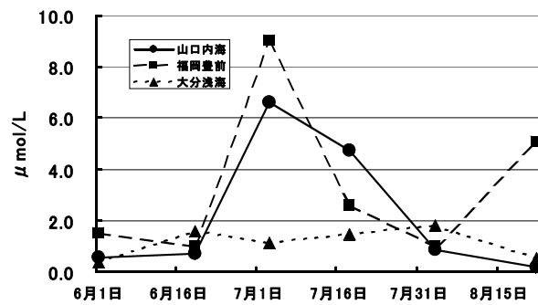
図10 DINの推移と全珪藻細胞数との関係
