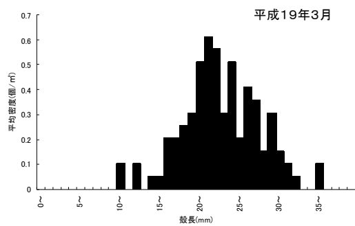
図3 蕨島干潟におけるアサリ殻長組成
