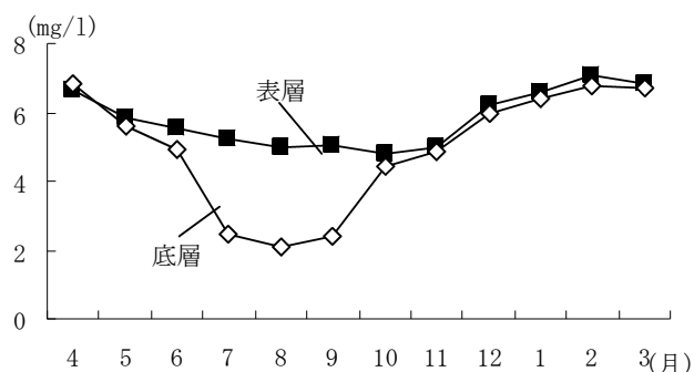
図5 溶存酸素の推移
