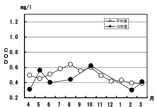
図5 CODの変化
