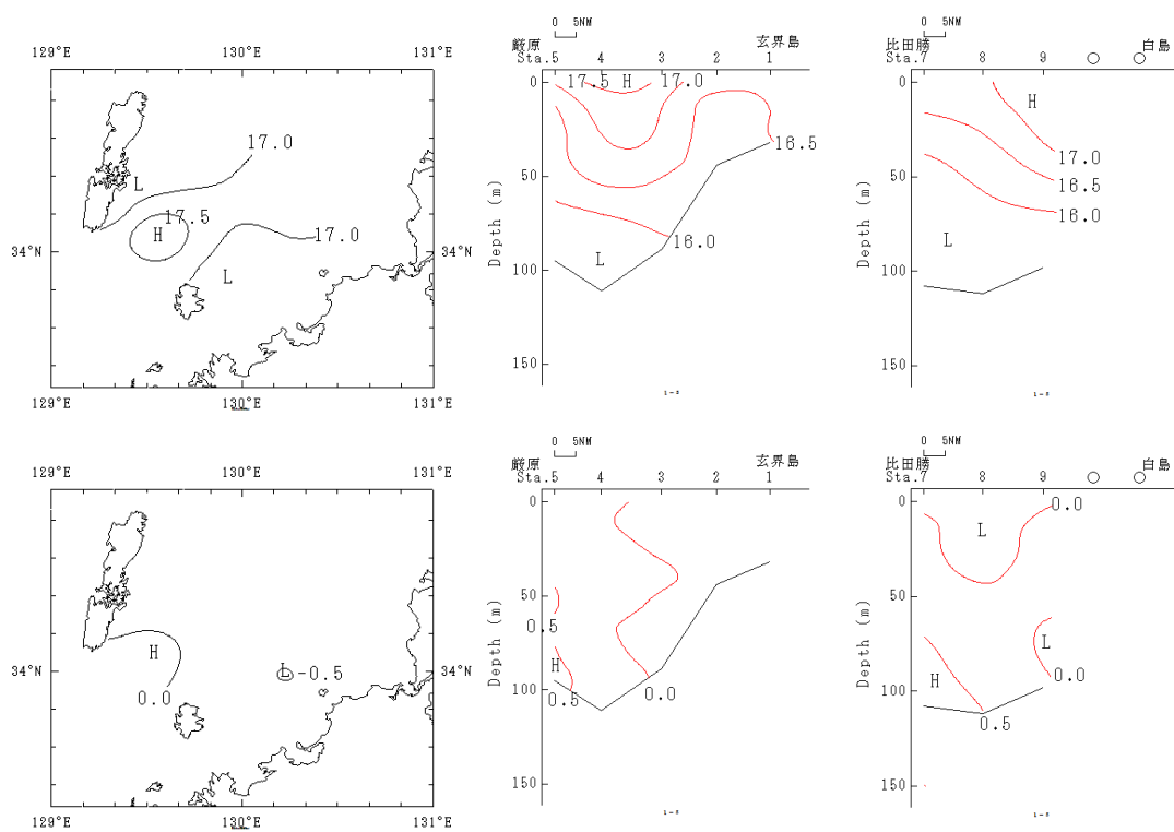
図2-① 水温の水平分布（表層）及び鉛直分布 (上段:実測値 下段:平年偏差)
