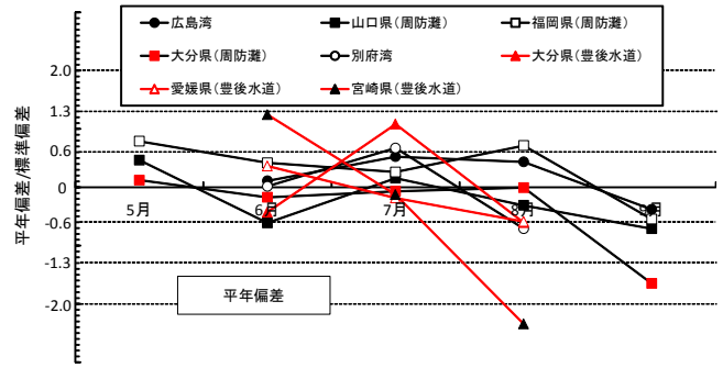
図13 各海域の溶存酸素飽和度最低値と平均値の年平均偏差
