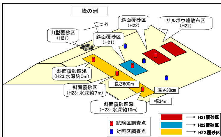
図2 覆砂工事概要図
