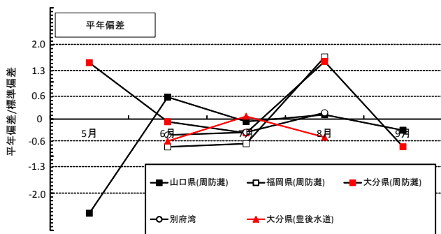
図12 各海域のクロロフィルaの平均値と年平均偏差
