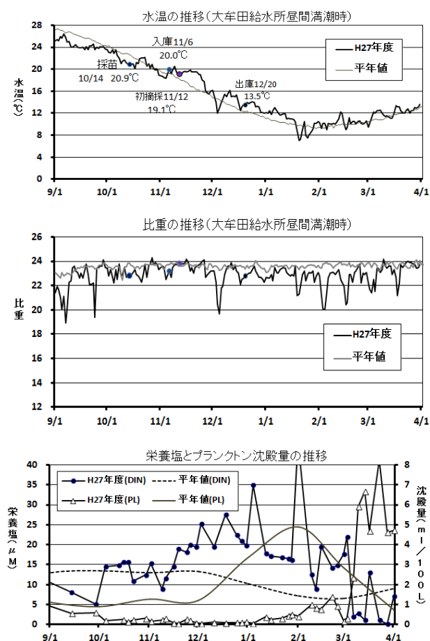
図 3 平成 27 年度ノリ漁期における水温、比重、栄養塩量及びプランクトン沈殿量の推移 (水温・比重の平年値：過去 30 年間の平均値 (S56～H22)，栄養塩量・プランクトン沈殿量の平年値：過去 10 年の旬別平均値 (H13～H22))
