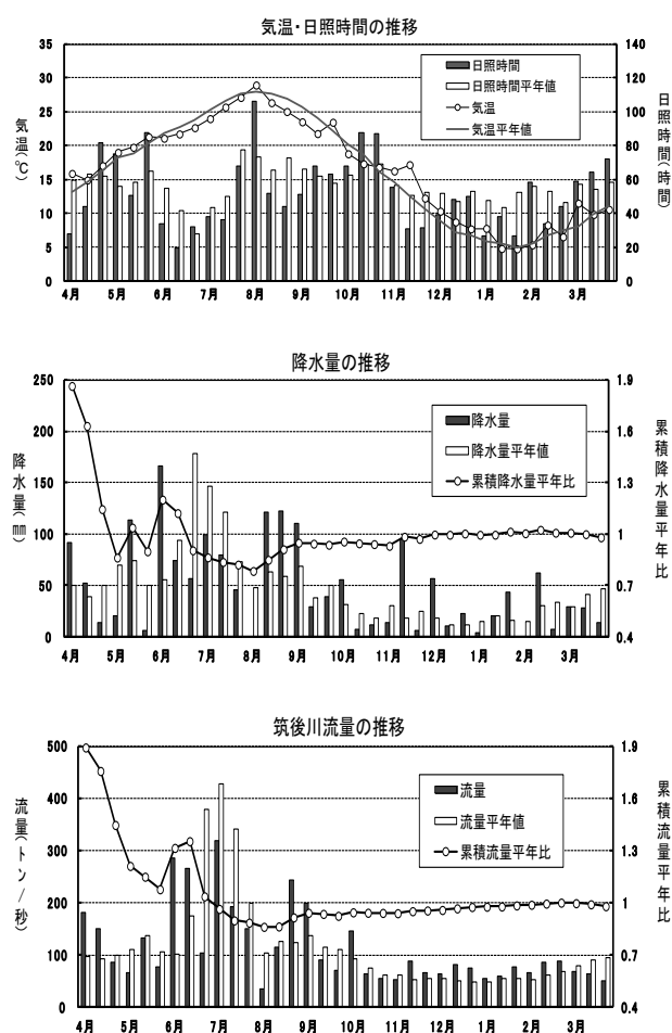
図 2 平成 27 年度ノリ漁期における気温、日照時間、降水量及び筑後川流量の推移 (平年値：過去 30 年間の平均値 (S56～H22))
