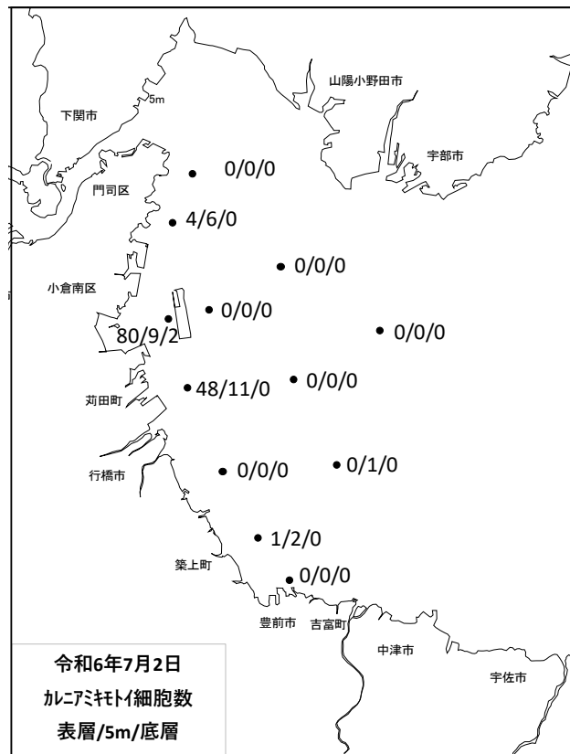
図 2 カレニア ミキモトイの細胞数（海水 1 cc あたり） ※数字は 0m/5m 層/B-1m 層の細胞数を示しています
