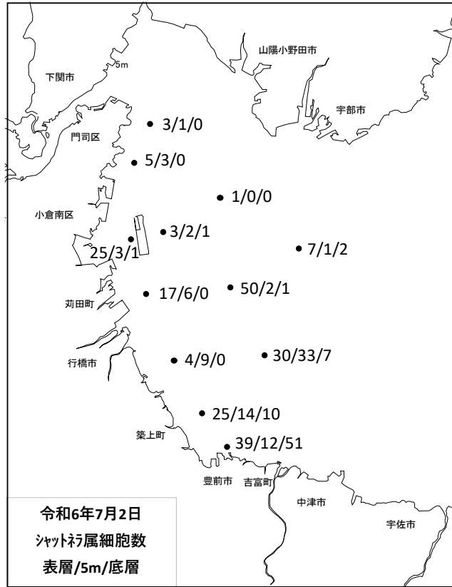
図 1 シャットネラ属の細胞数（海水 1 cc あたり）
