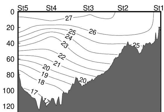
厳原～玄界島 垂直分布
