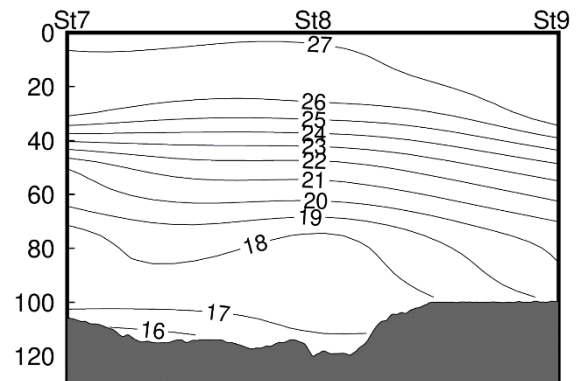
比田勝～沖島東 垂直分布
